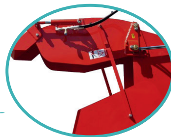
Vérin hydraulique sur casquette de goulotte
