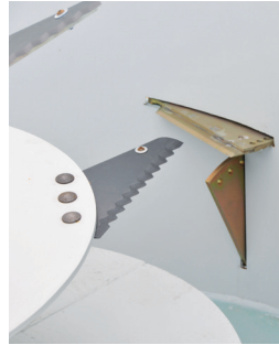
UN CONTRE-COUTEAU VERTICAL ET UN CONTRE-COUTEAU HORIZONTAL POUR AMÉLIORER LA VITESSE DE COUPE
