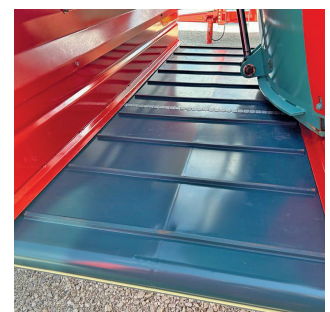
TAPIS BILATÉRAL PVC À PLAT UNIQUEMENT, LARGEUR 800 MM EN REMPLACEMENT DES CHAÎNES ET BARRETTES
